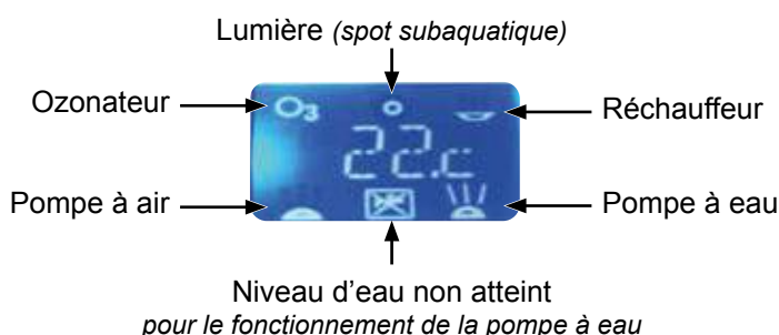
Écran LCD
